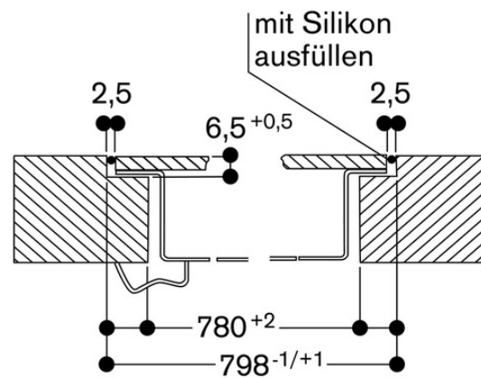
Längsschnitt
